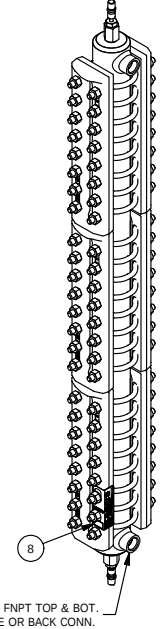
TRANSPARENT GAGE TTLCH-10
